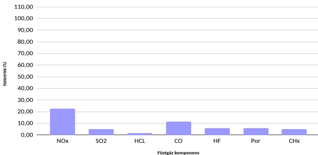
A SARPI Dorog Kft. 2022. évi átlag emissziós adatai a 29/2014. FM rendelet féllóras határértékeinek százalékában
